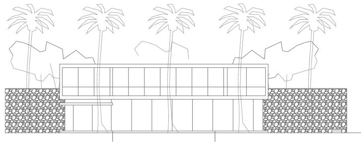
Alzado Oeste/West Elevation
