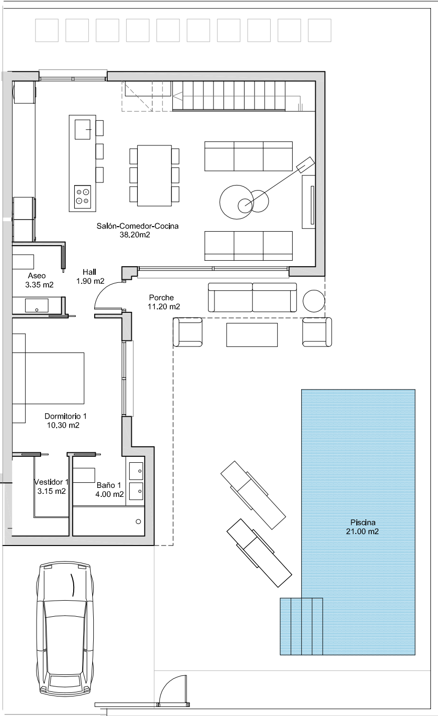
Planta baja
