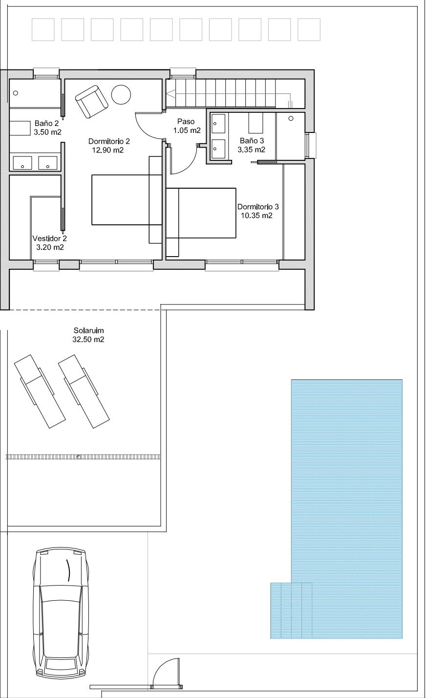
Planta primera
