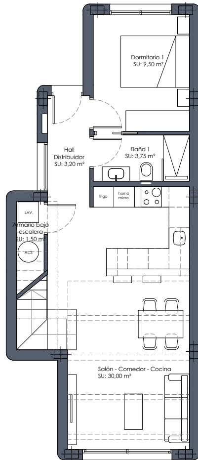
PLANTA BAJA
