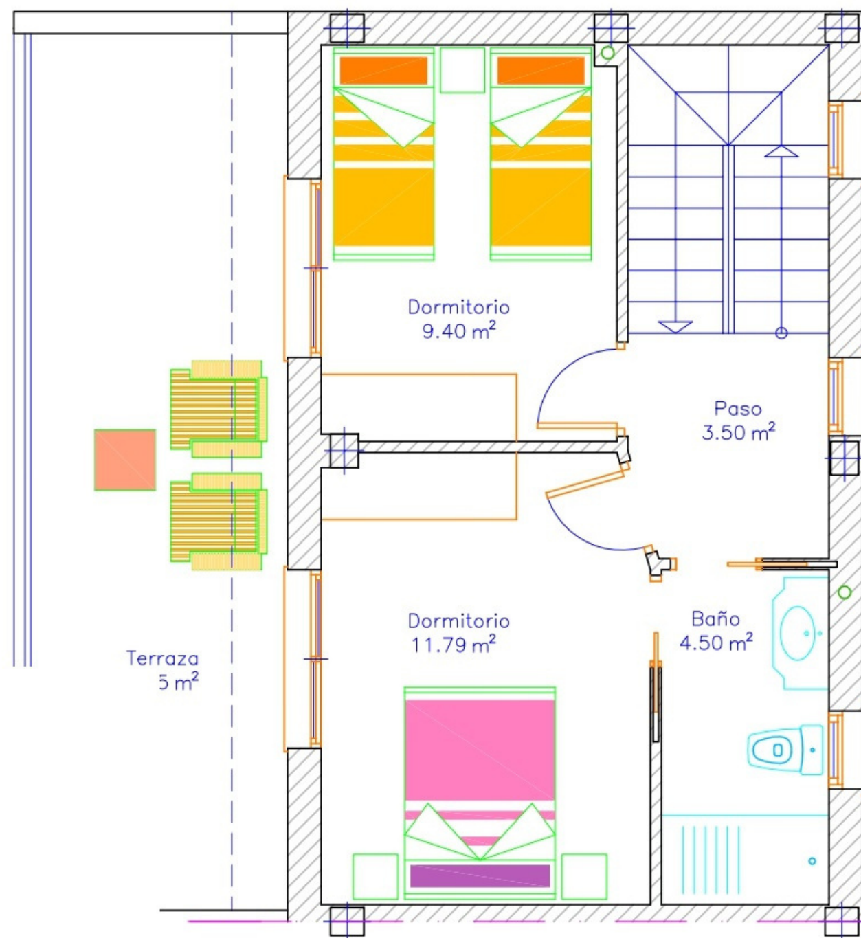
PLANTA 1, S.C.= 44.01M2
