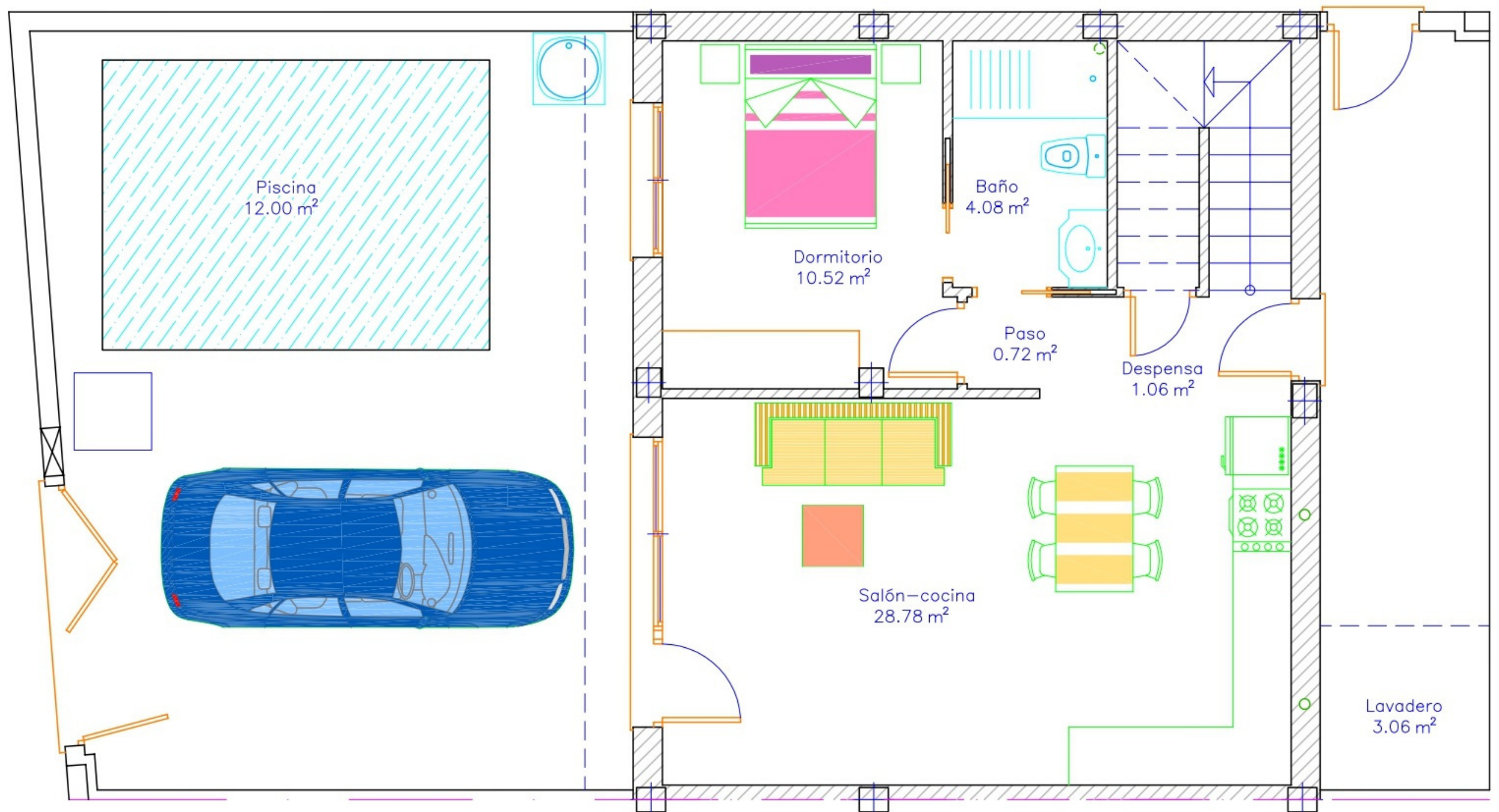
PLANTA 0, S.C.= 63.14M2
