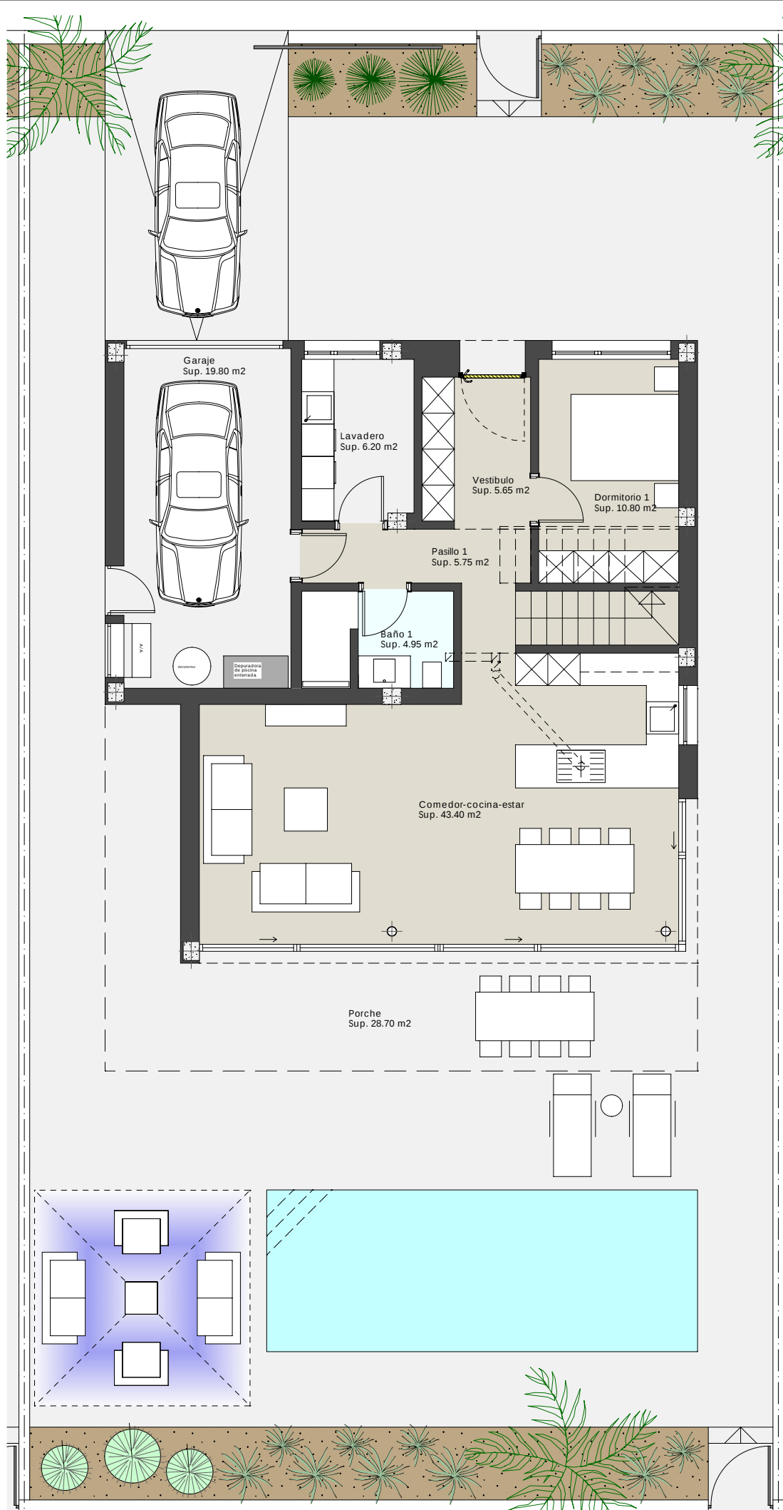
PLANTA BAJA
