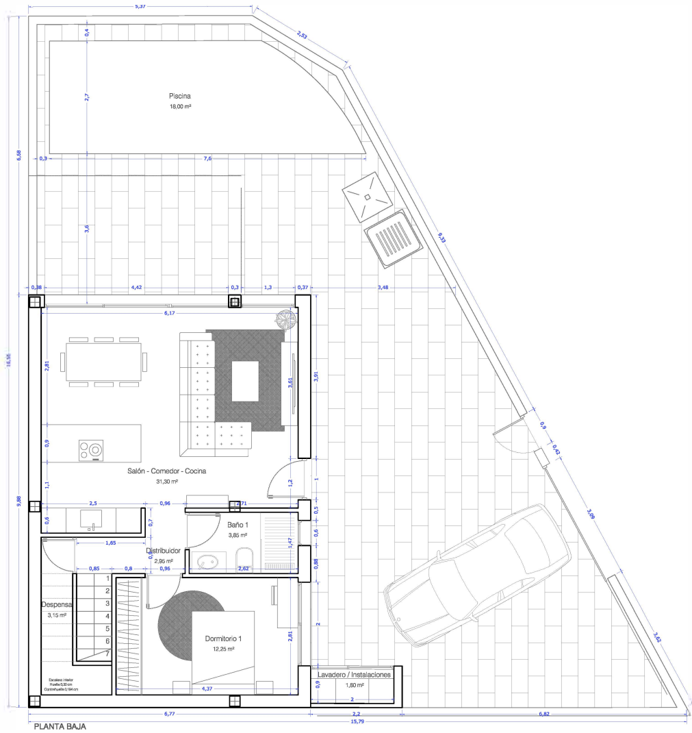
PLANTA BAJA
