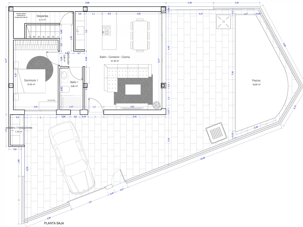
PLANTA BAJA
