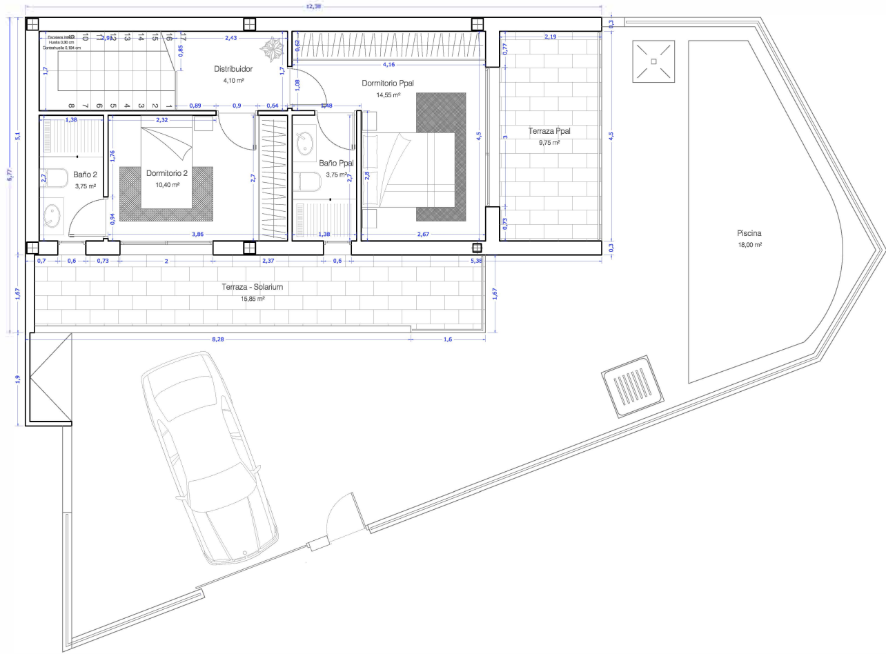
PLANTA PRIMERA
