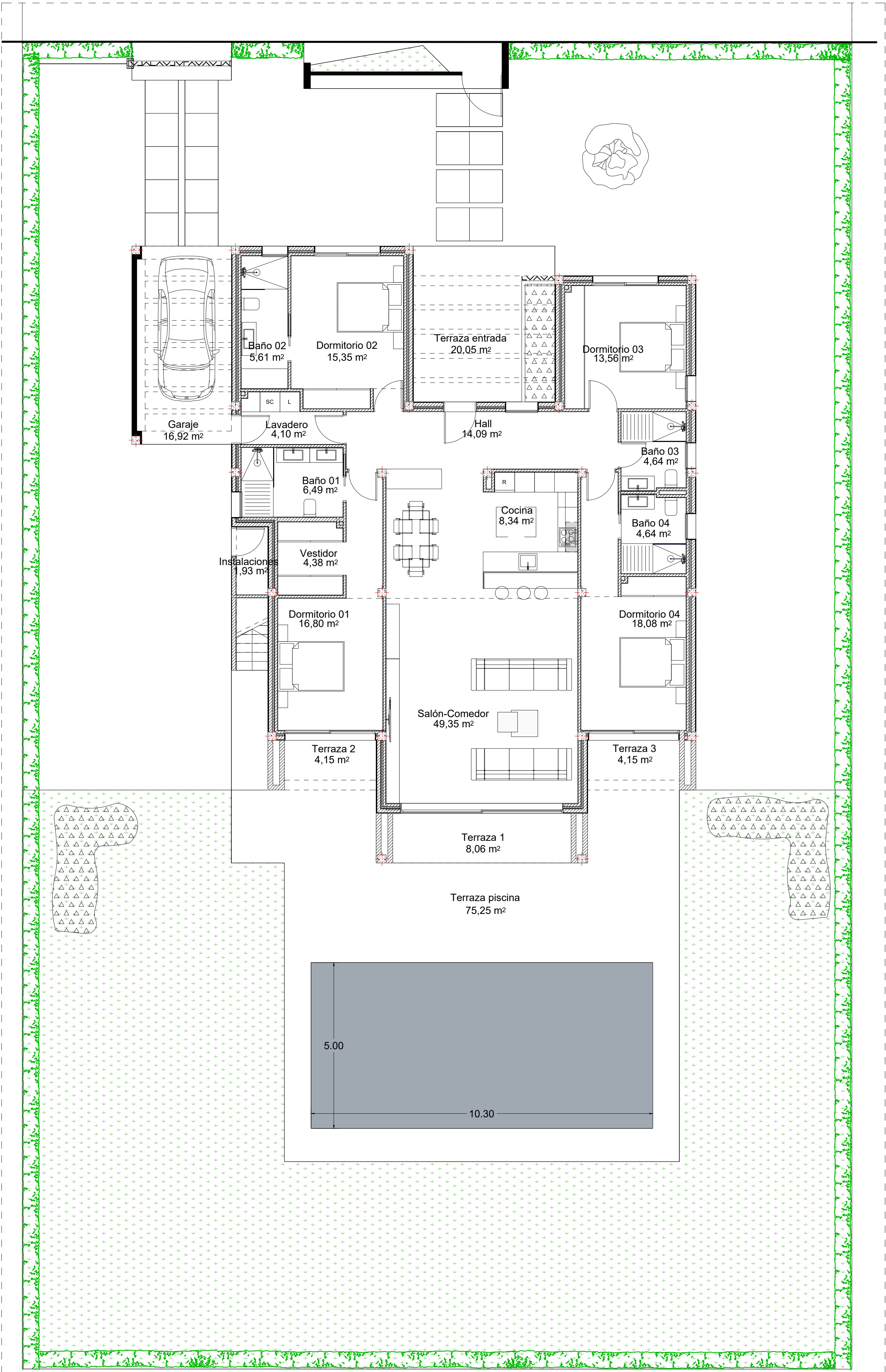
Planta Baja
