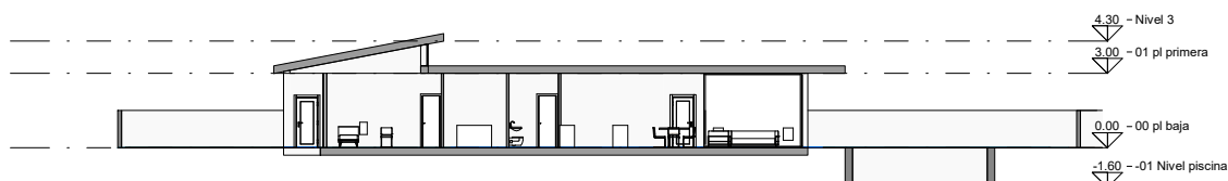
4 Sección 1 001 1 : 150
