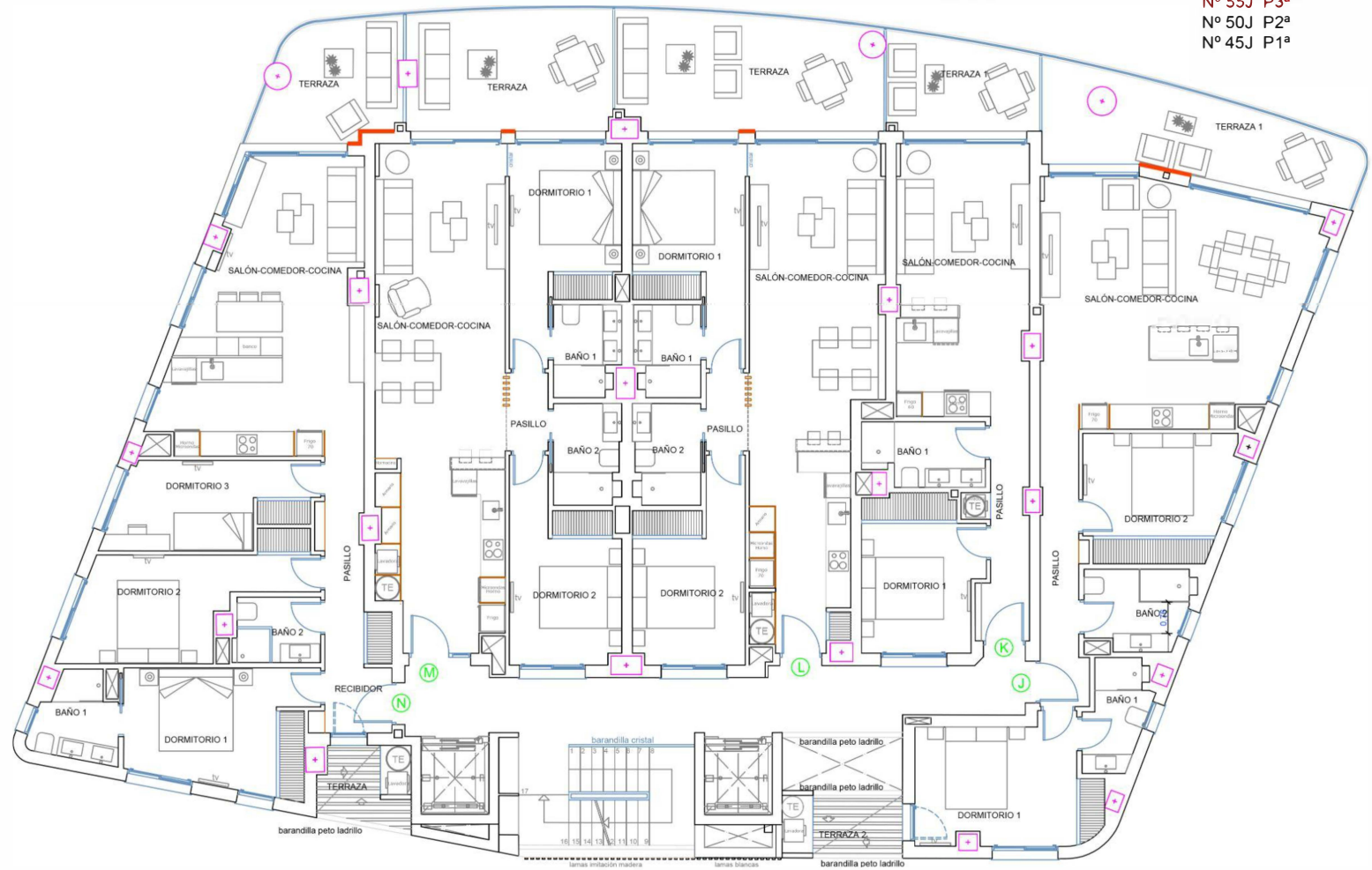
Bloque B - Plantas 1ª, 2ª, 3ª, 4ª, 5ª, 6ª, 7ª y 8ª
