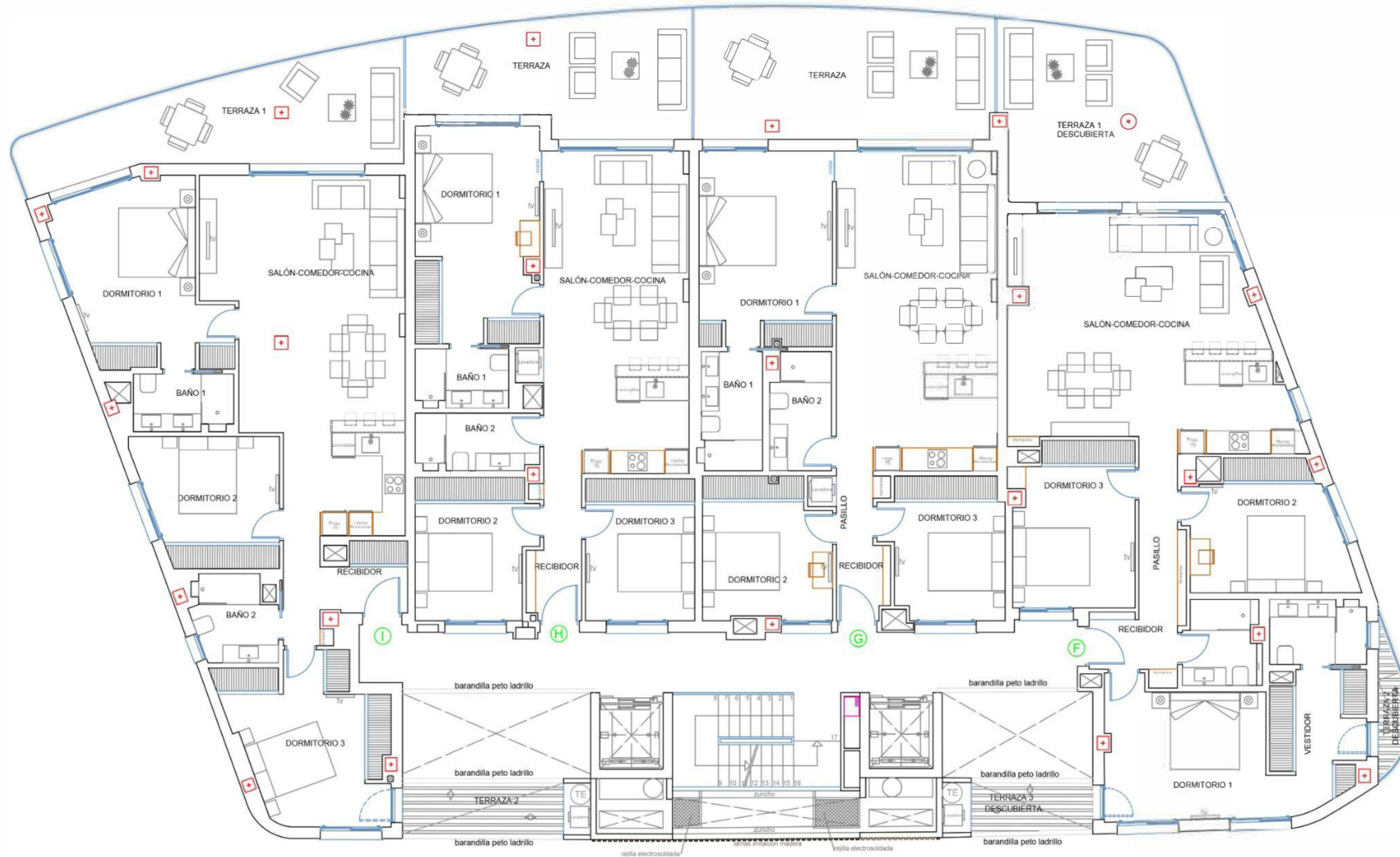
Bloque A - Planta 9ª (Atico)
