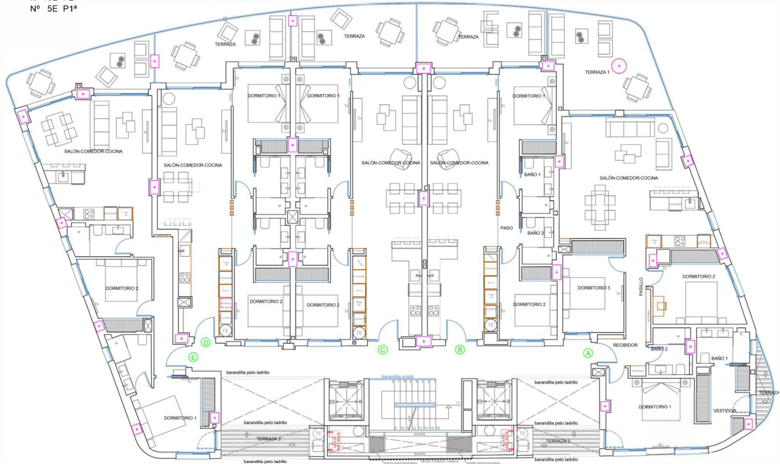
Bloque A - Plantas 1ª, 2ª, 3ª, 4ª, 5ª, 6ª, 7ª y 8ª
