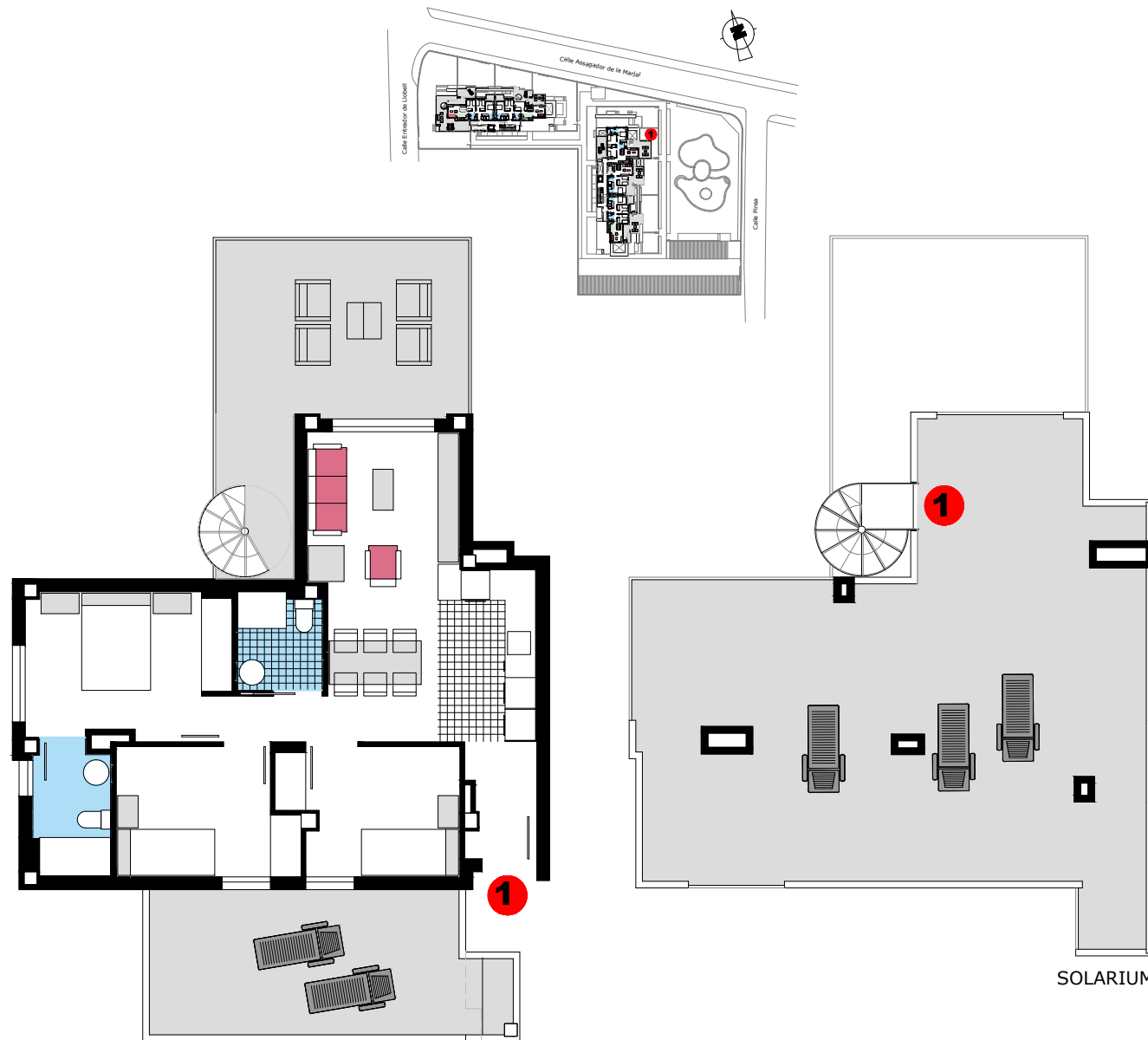
PLANTA ATICO - ESCALERA B
