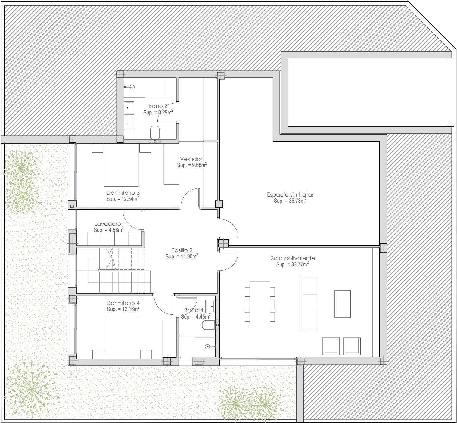
Planta inferior
