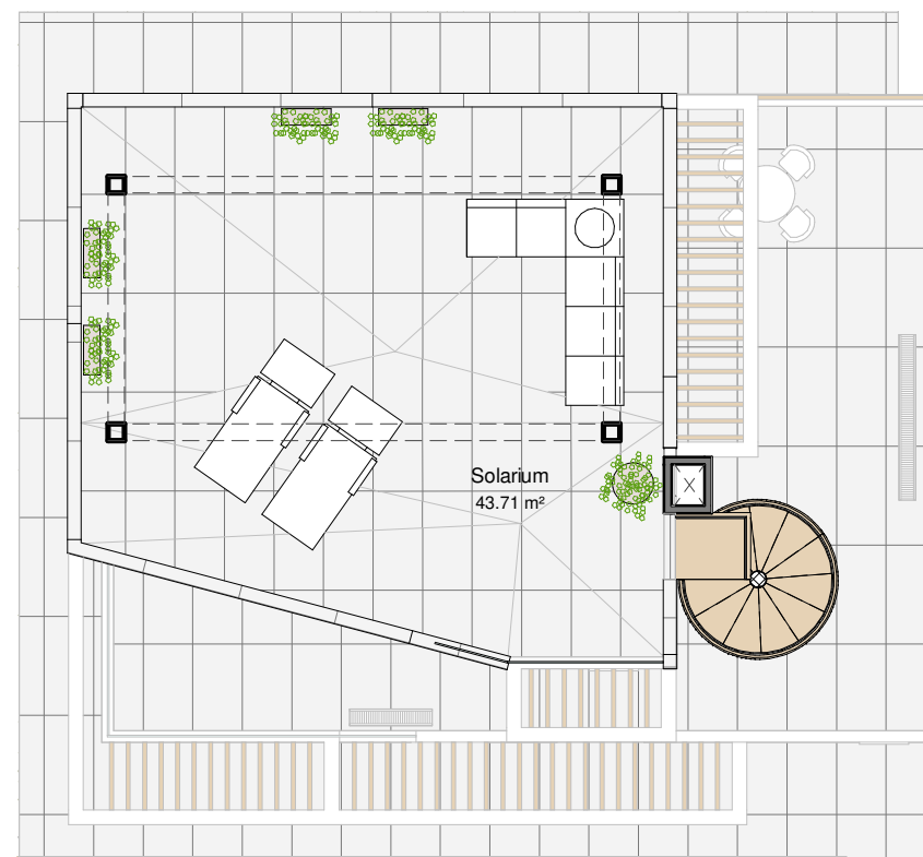
PLANTA CUBIERTA
