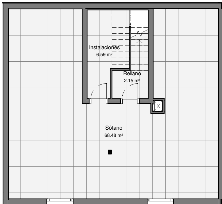
PLANTA SÓTANO
