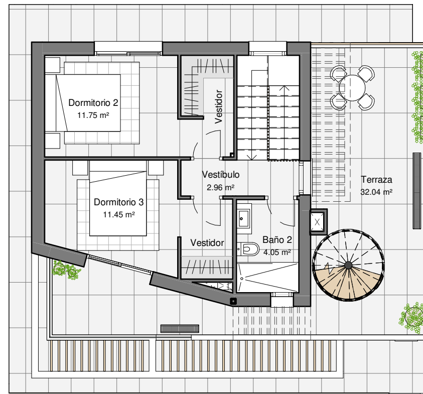
PLANTA PRIMERA
