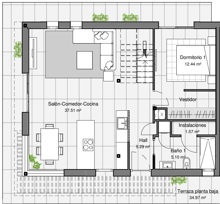
PLANTA BAJA
