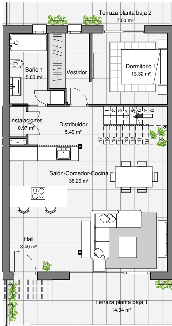
PLANTA BAJA
