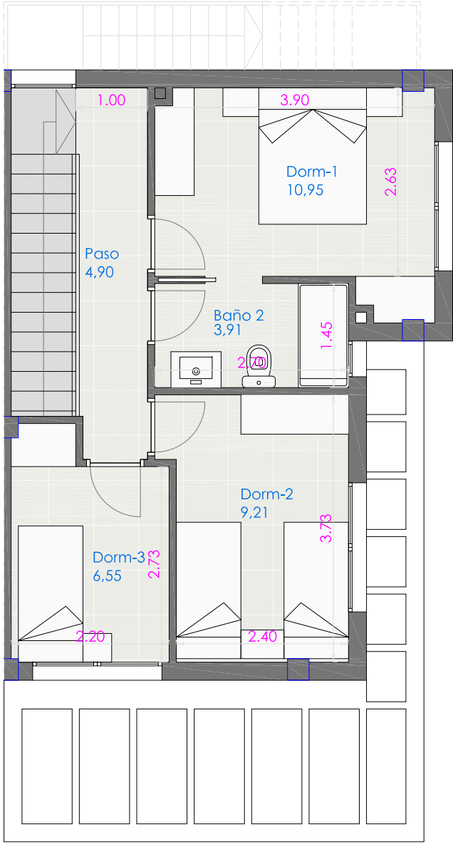
PLANTA ALTA
