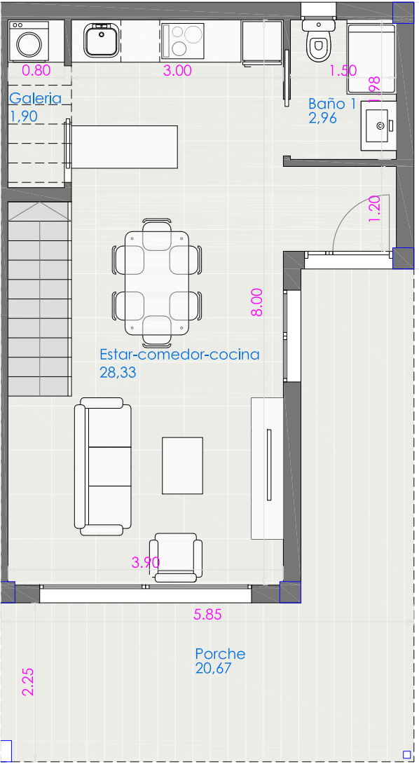
PLANTA BAJA
