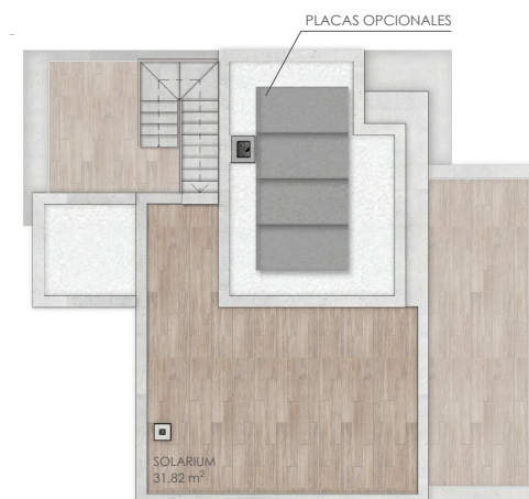
PLANTA SOLARIUM
