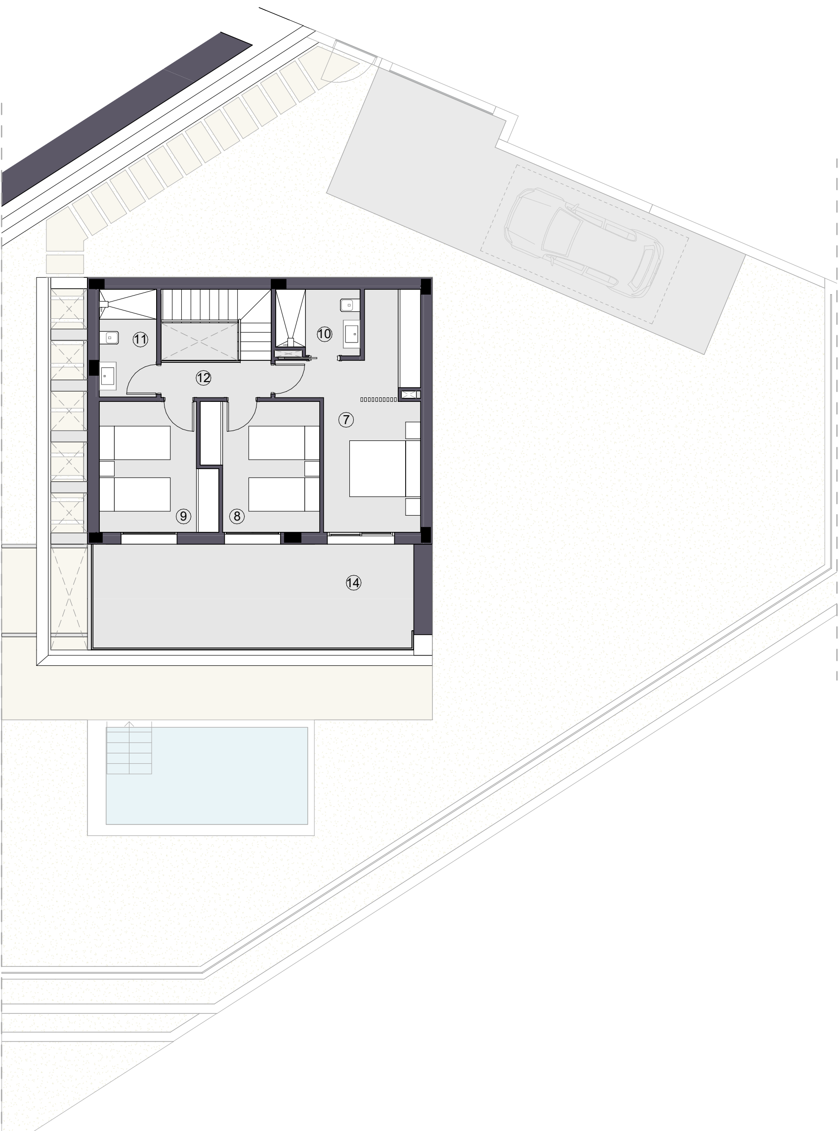
PLANTA PRIMERA / FIRST FLOOR
