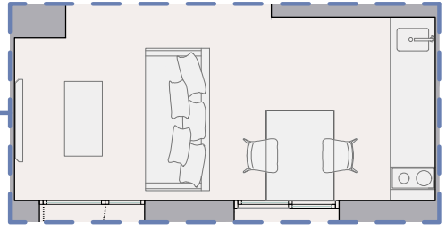
Opción 2: Living + kichenette Planta / Floor Inferior
