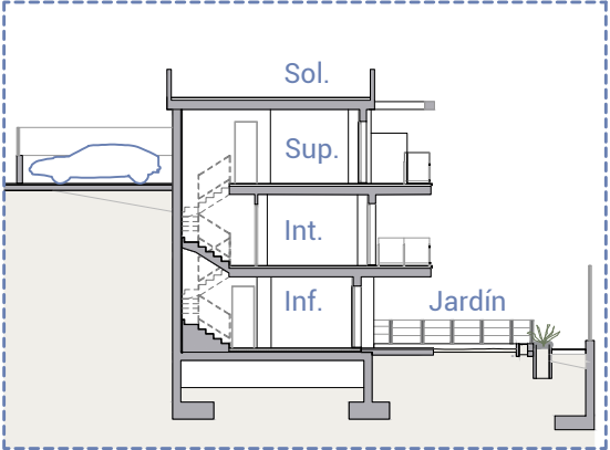
Sección / Section
