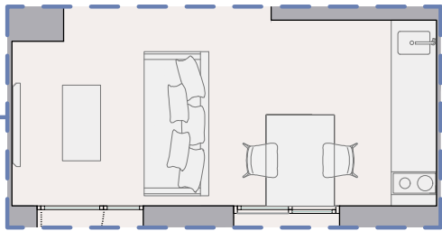
Opción 2: Living + kichenette Planta / Floor Inferior
