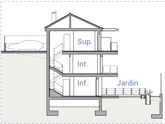
Sección / Section
