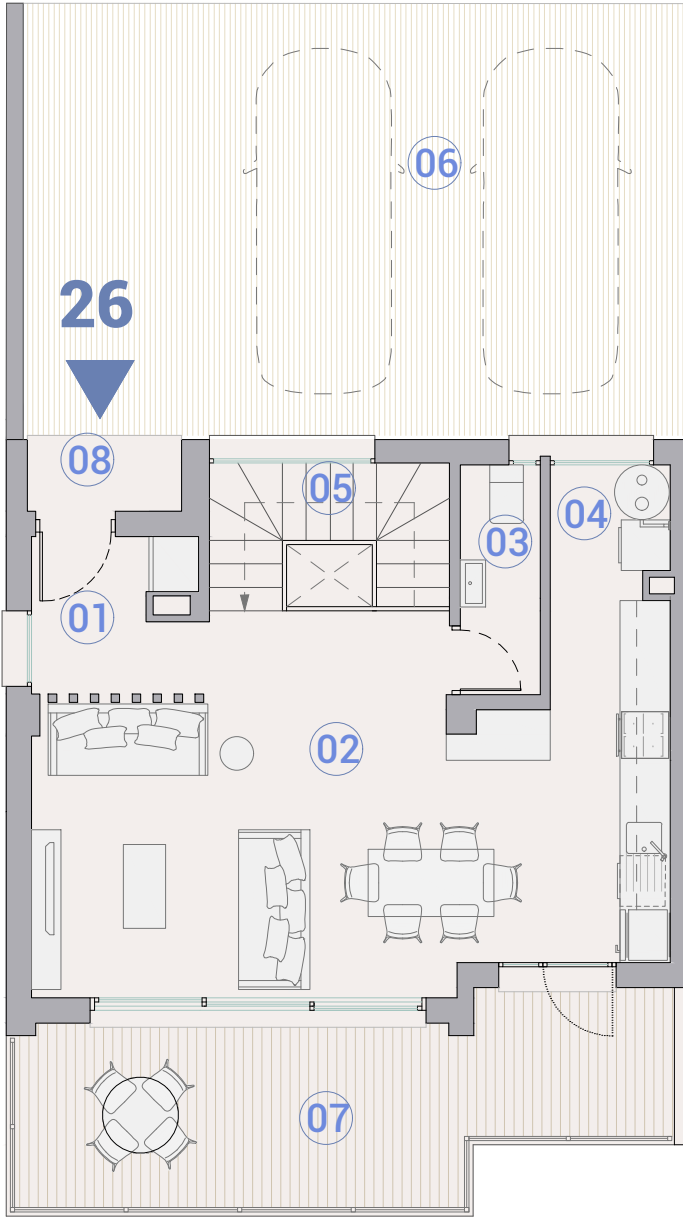
Planta / Floor Superior
