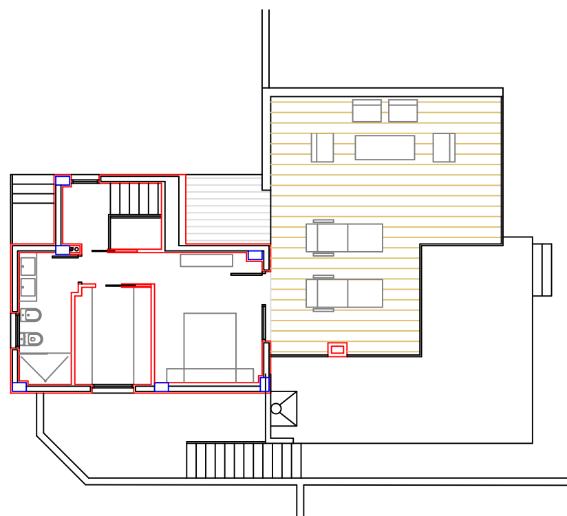
PLANTA PISO
