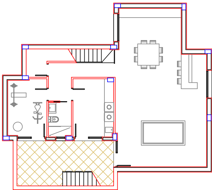
PLANTA SEMISOTANO
