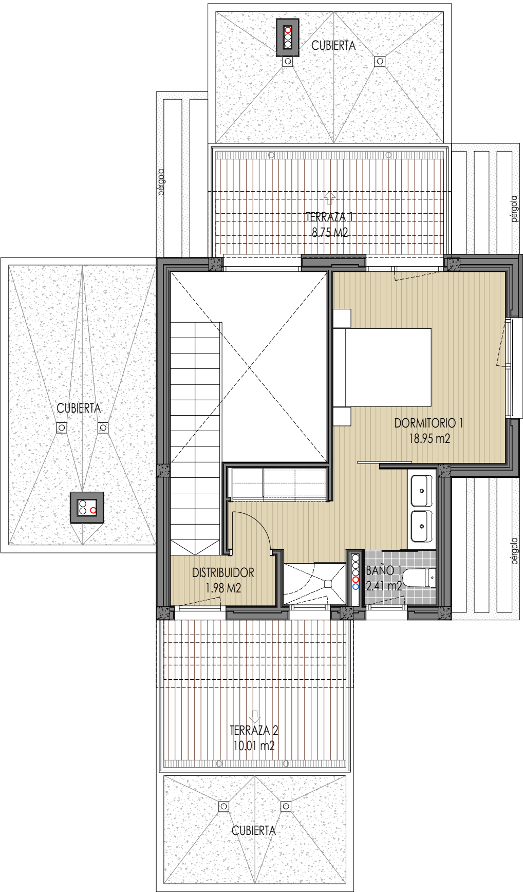
PLANTA PRIMERA
