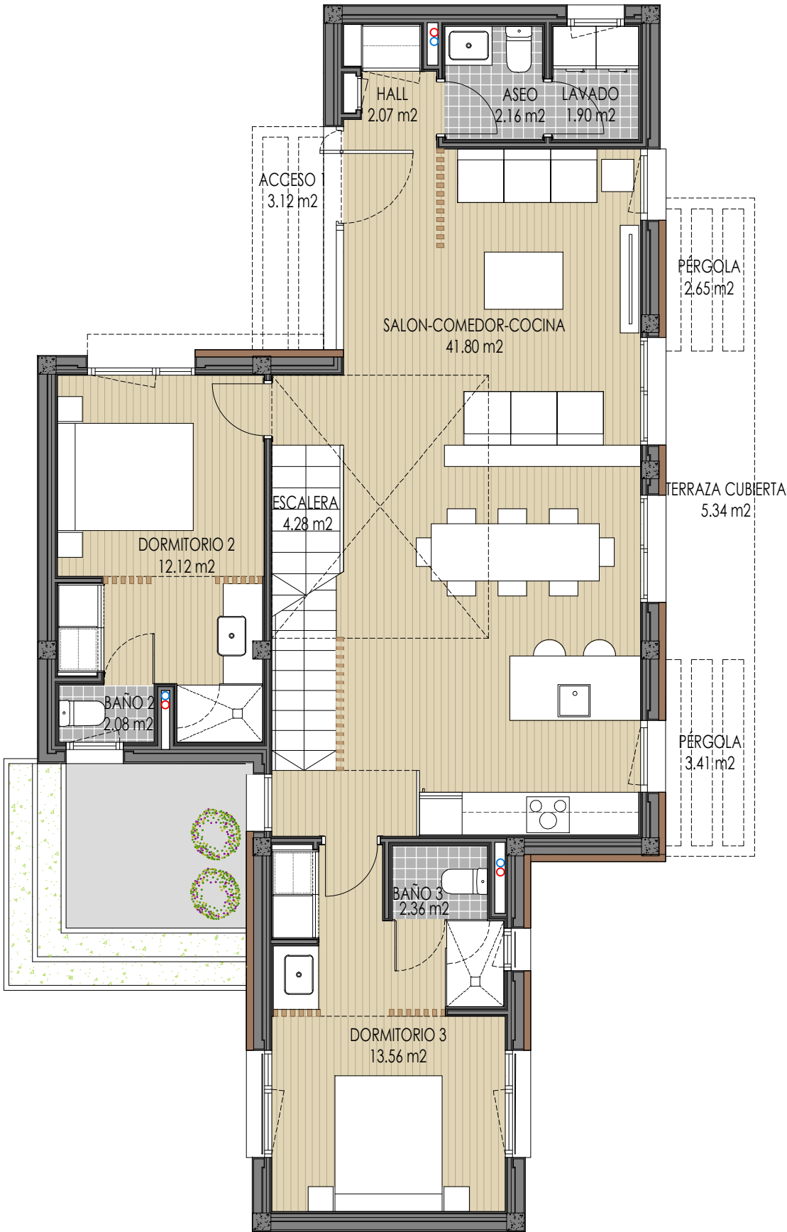
PLANTA BAJA
