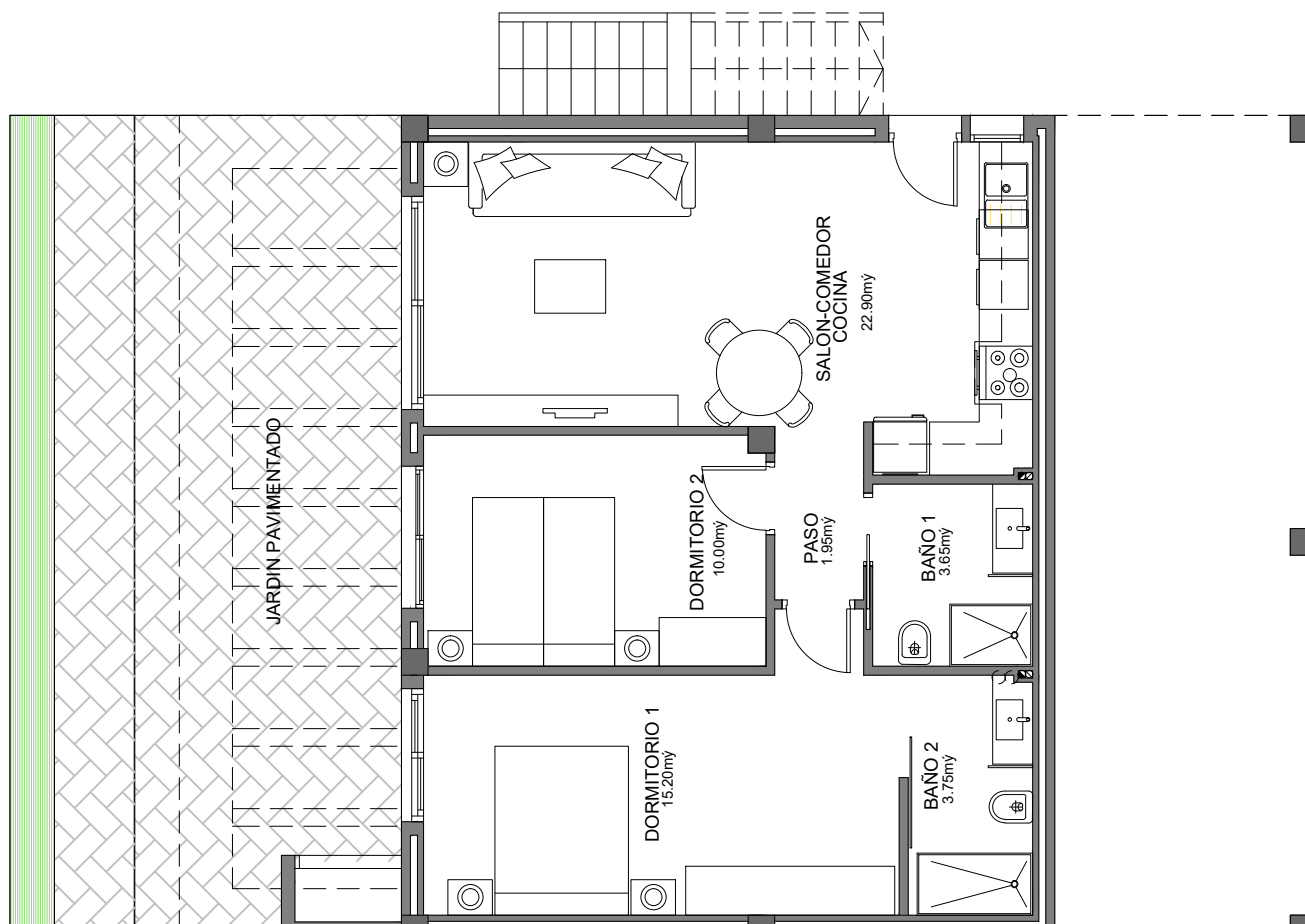
Planta Baja
