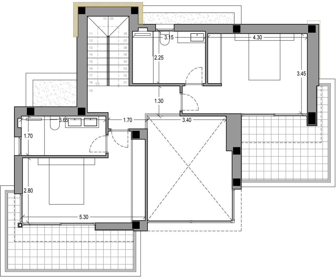
PLANTA ALTA - COTAS
