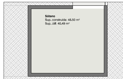
PLANTA SÓTANO
