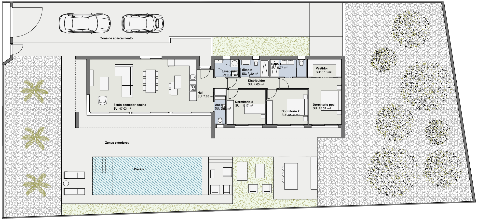
PLANTA BAJA
