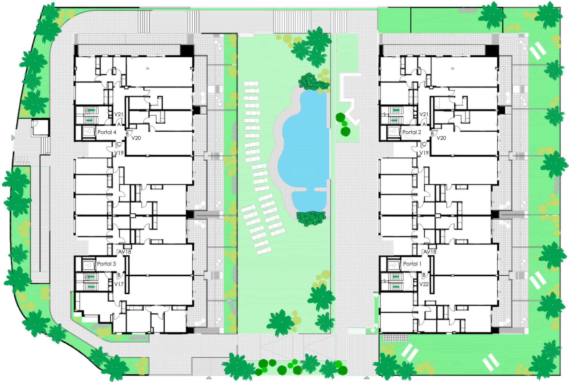
PLANTA TERCERA
