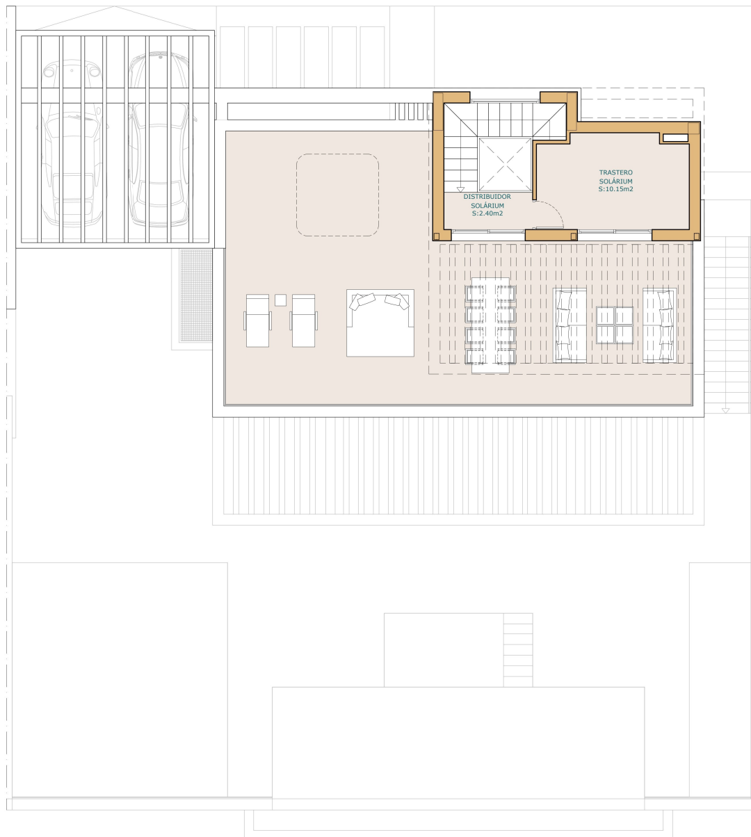
PLANTA SOLÁRIUM
