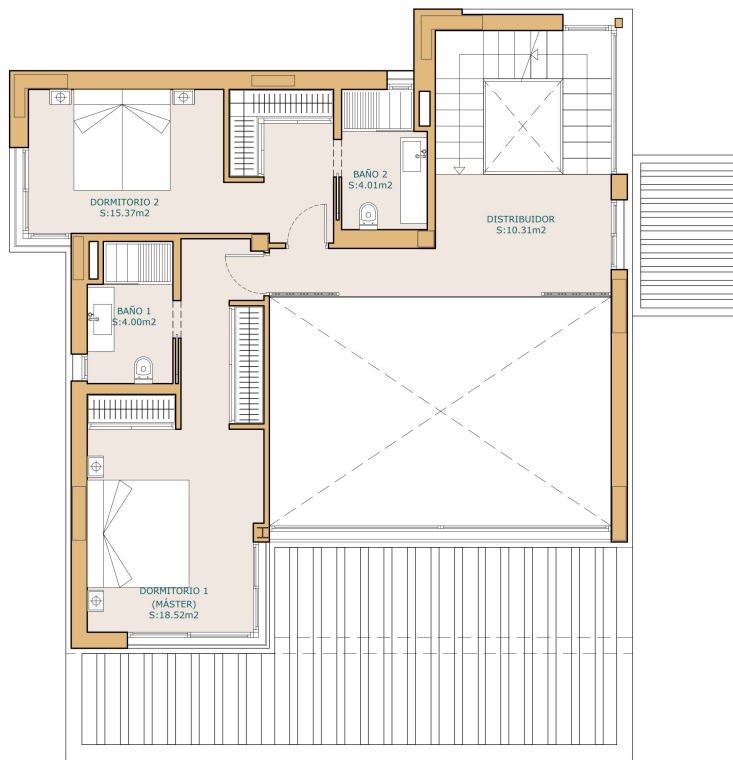
PLANTA PRIMERA
