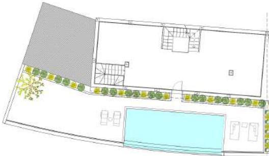
PLANTA -2
