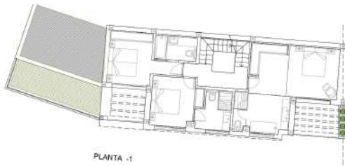
PLANTA -1
