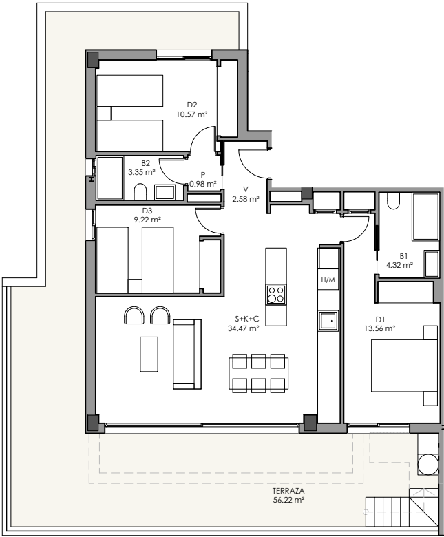
PLANTA TERCERA
