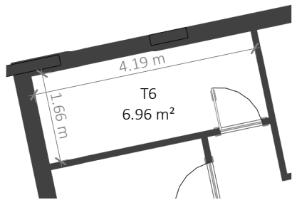
Planta Sótano 2 - zoom trastero 1 : 100 / S02 - STORAGE ROOM ZOOM
