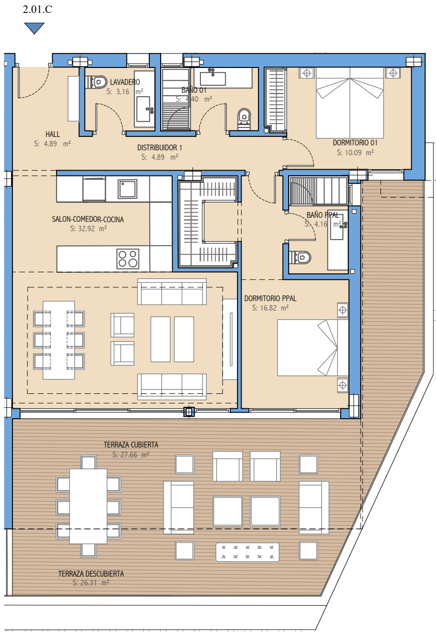
PLANTA PRIMERA
