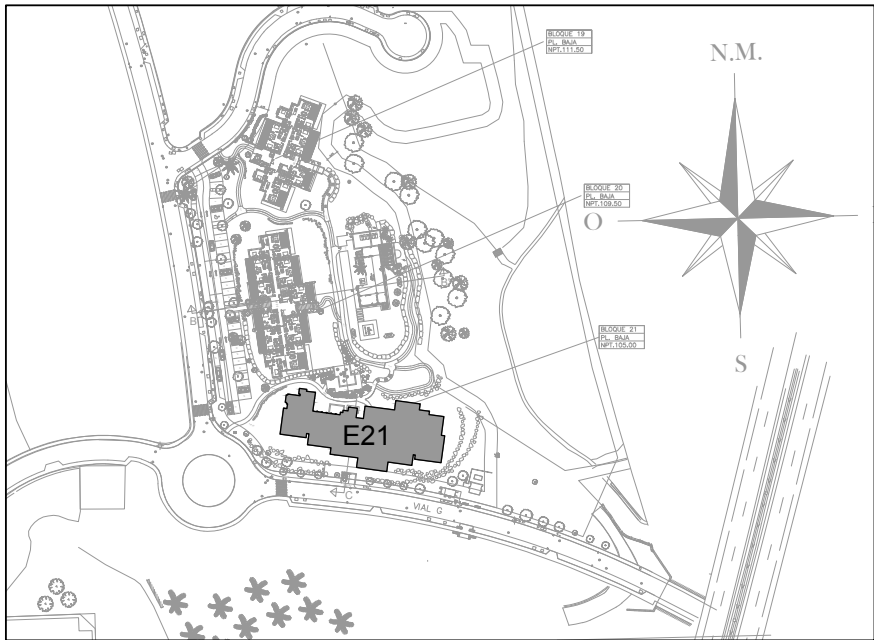
SITUACION GENERAL
