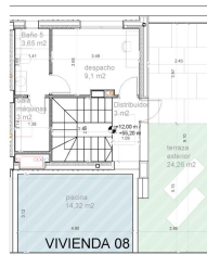
PLANTA SEGUNDA
