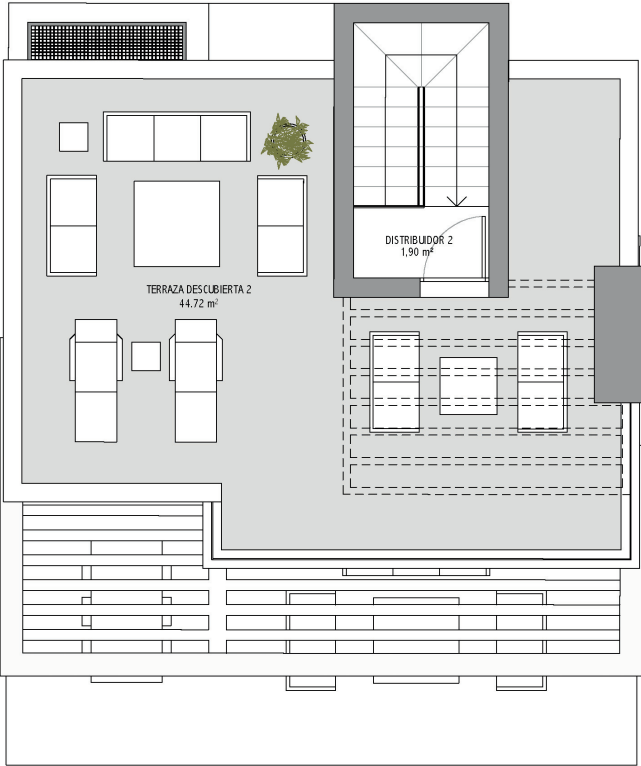
PLANTA SOLARIUM 1:75
