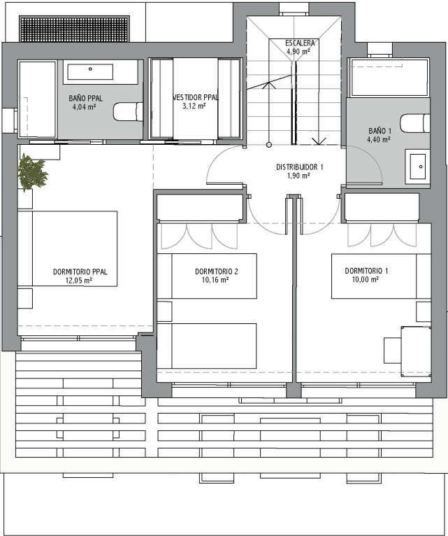
PLANTA ALTA 1:75
