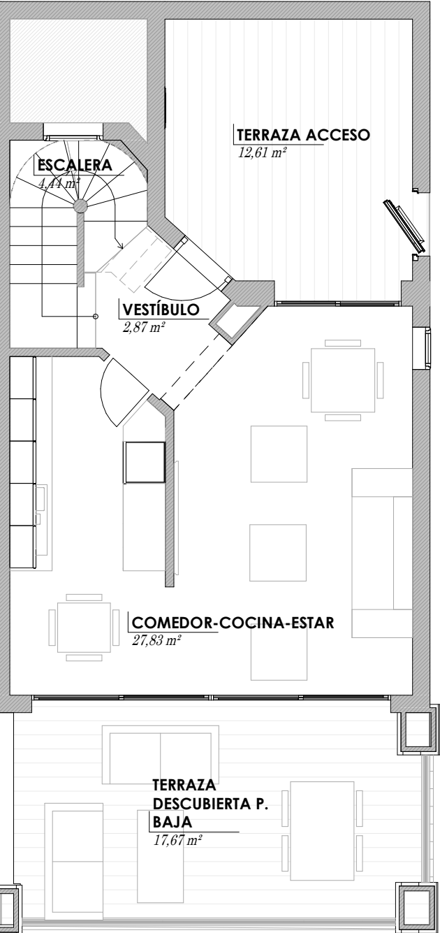
PLANTA BAJA
