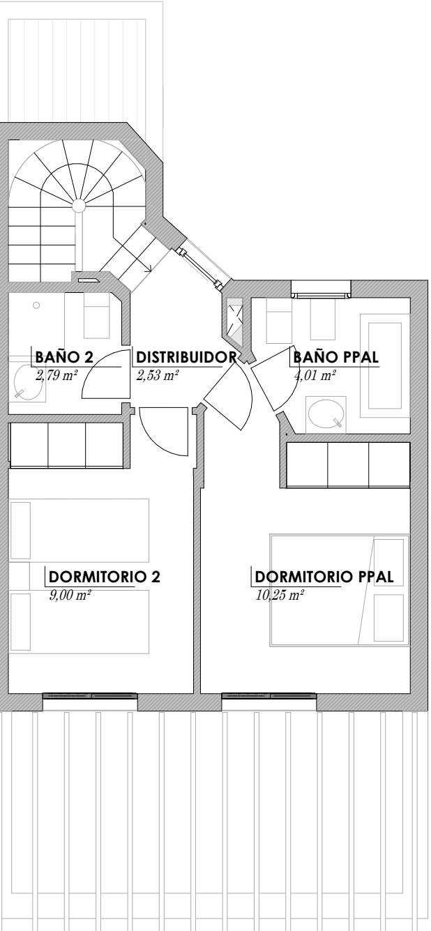
PLANTA PRIMERA
