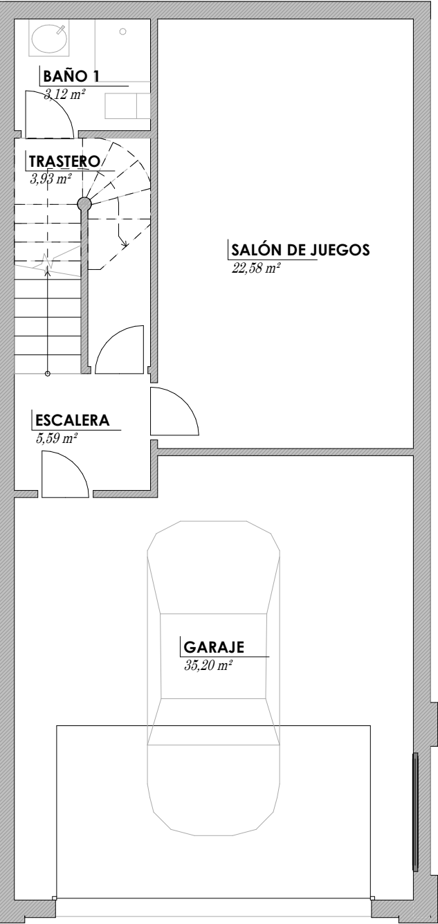
PLANTA SÓTANO
