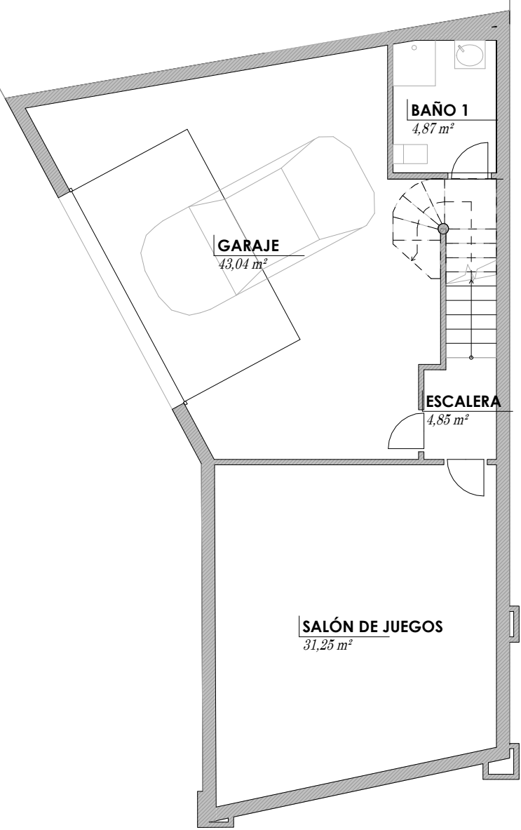
PLANTA SÓTANO
