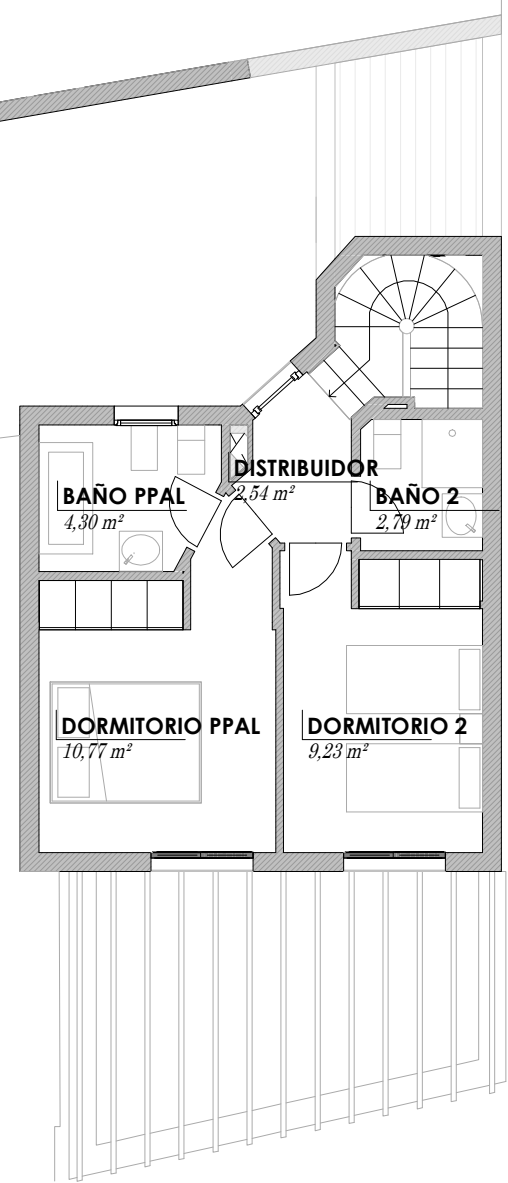
PLANTA PRIMERA
