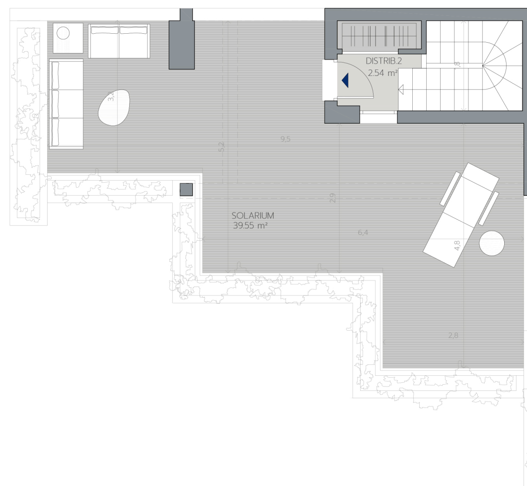
PLANTA SUPERIOR
