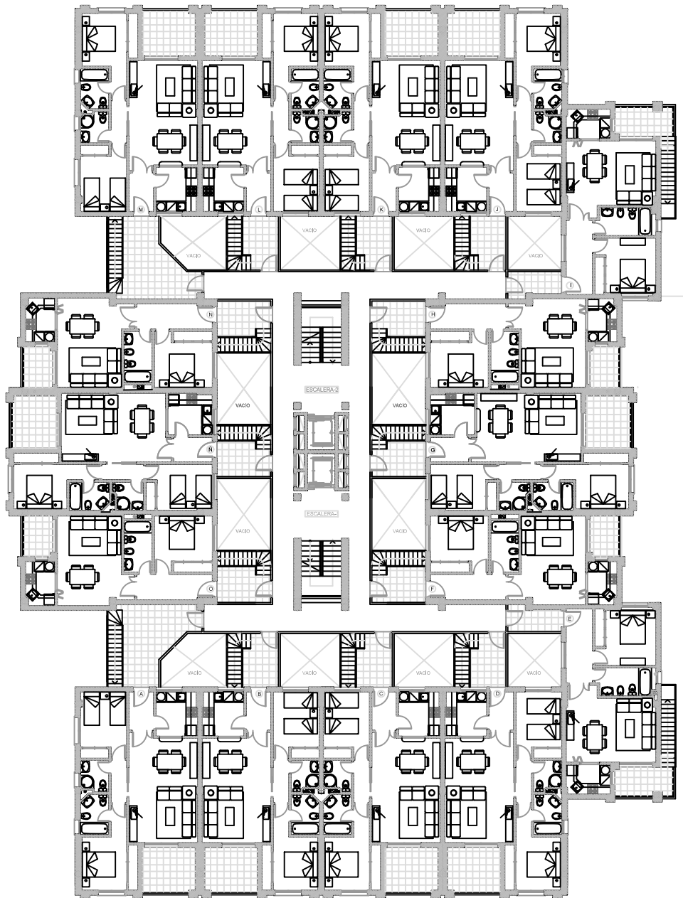
PLANTA TERCERA
