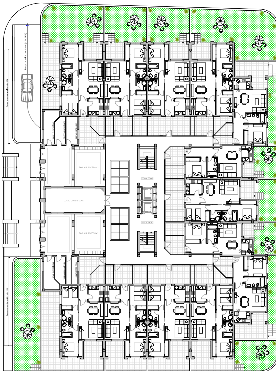
PLANTA BAJA
