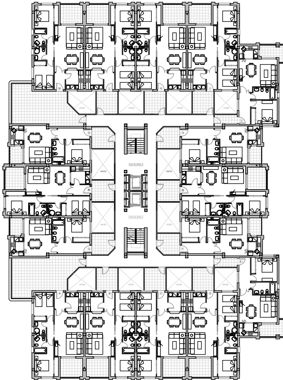
PLANTA PRIMERA
