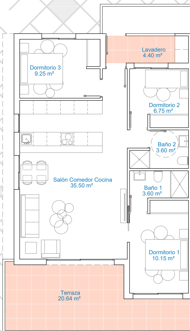
PLANTA PRIMERA
