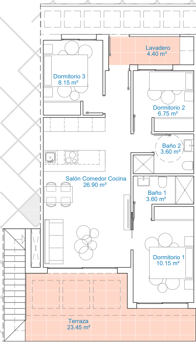
PLANTA ÁTICO
