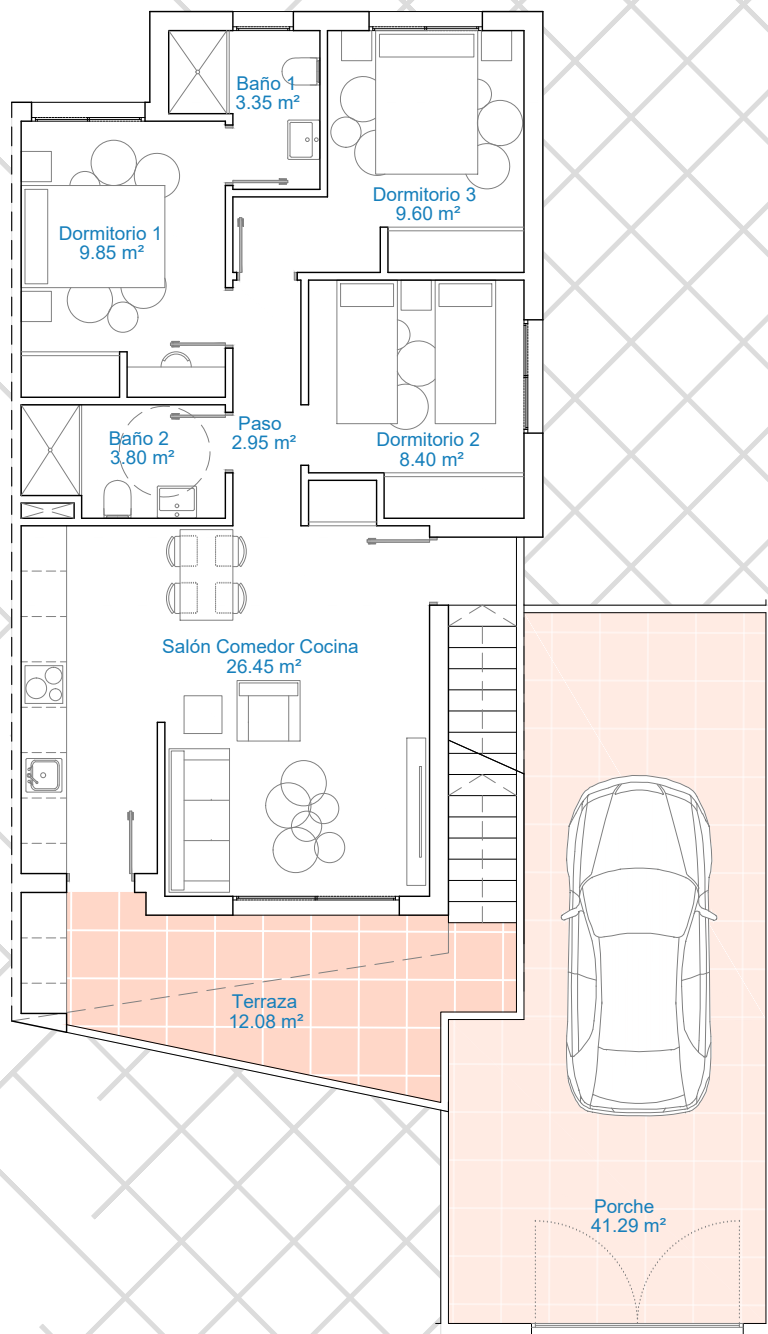
PLANTA PRIMERA
