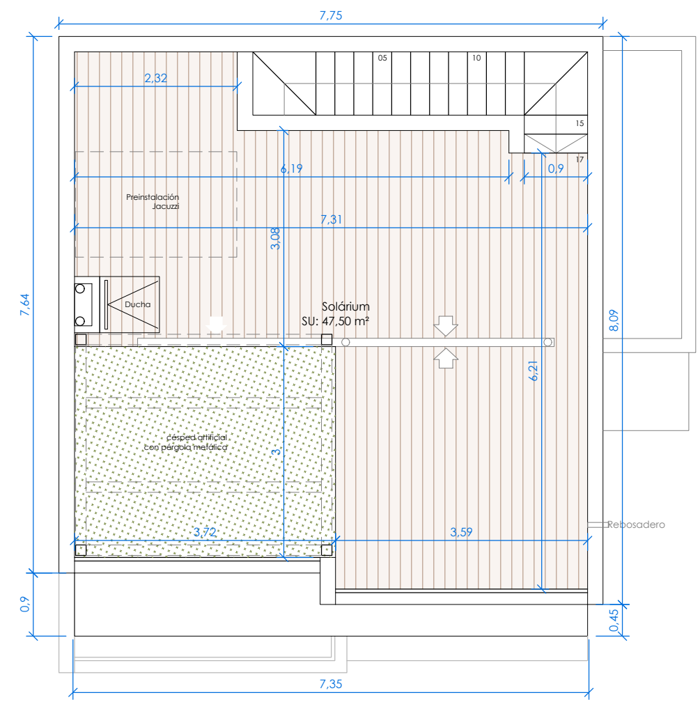
PLANTA CUBIERTA
