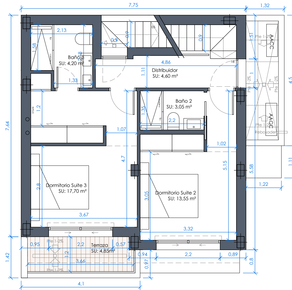
PLANTA PRIMERA
