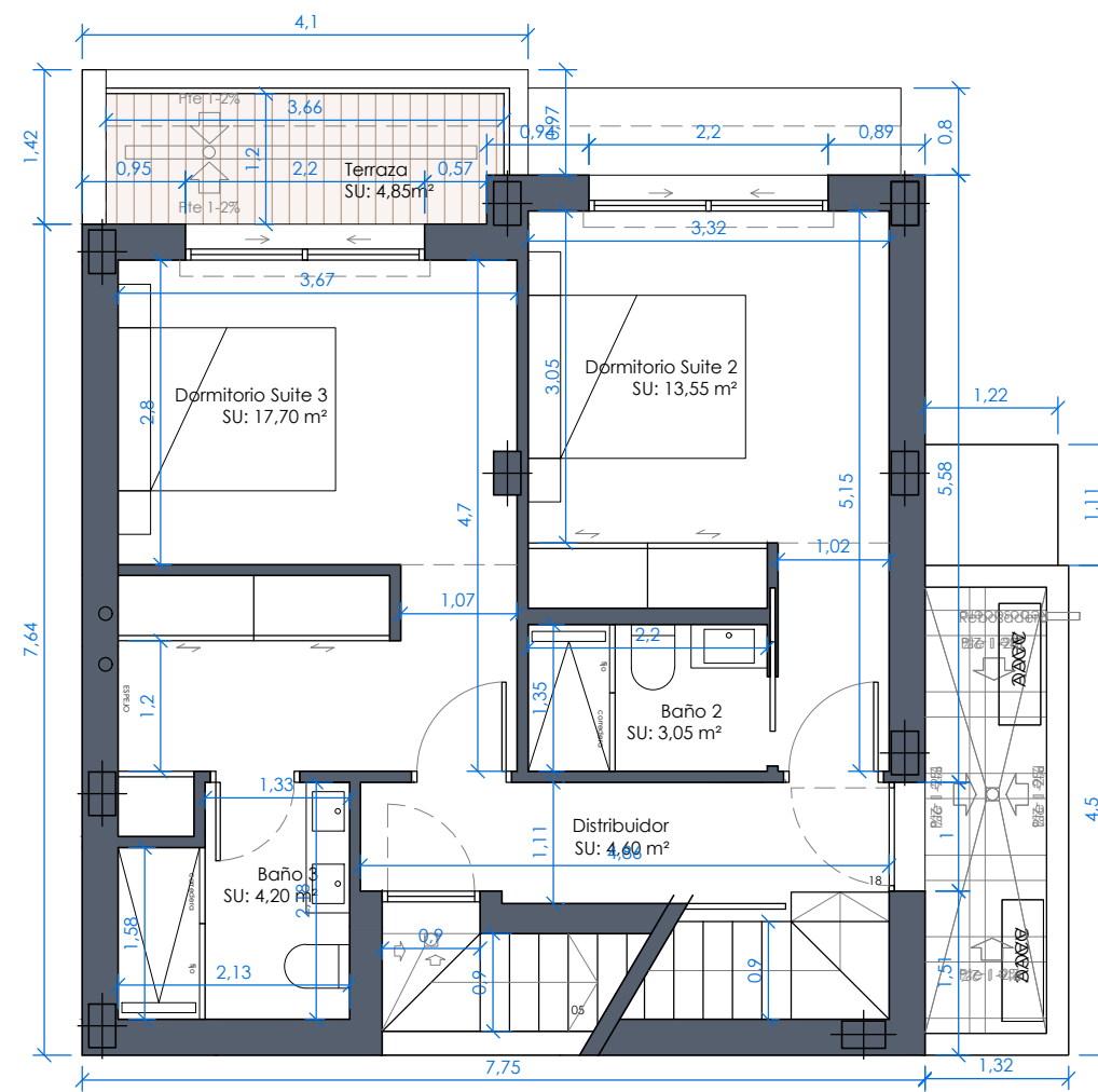
PLANTA PRIMERA
