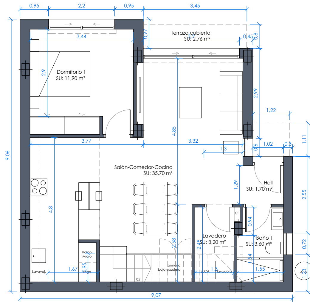
PLANTA BAJA
