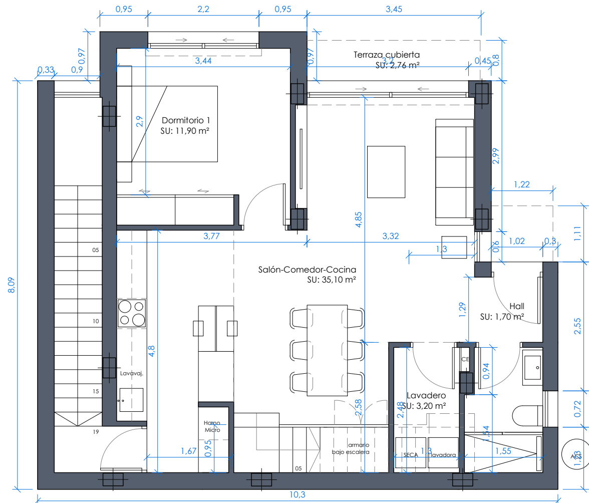
PLANTA BAJA
