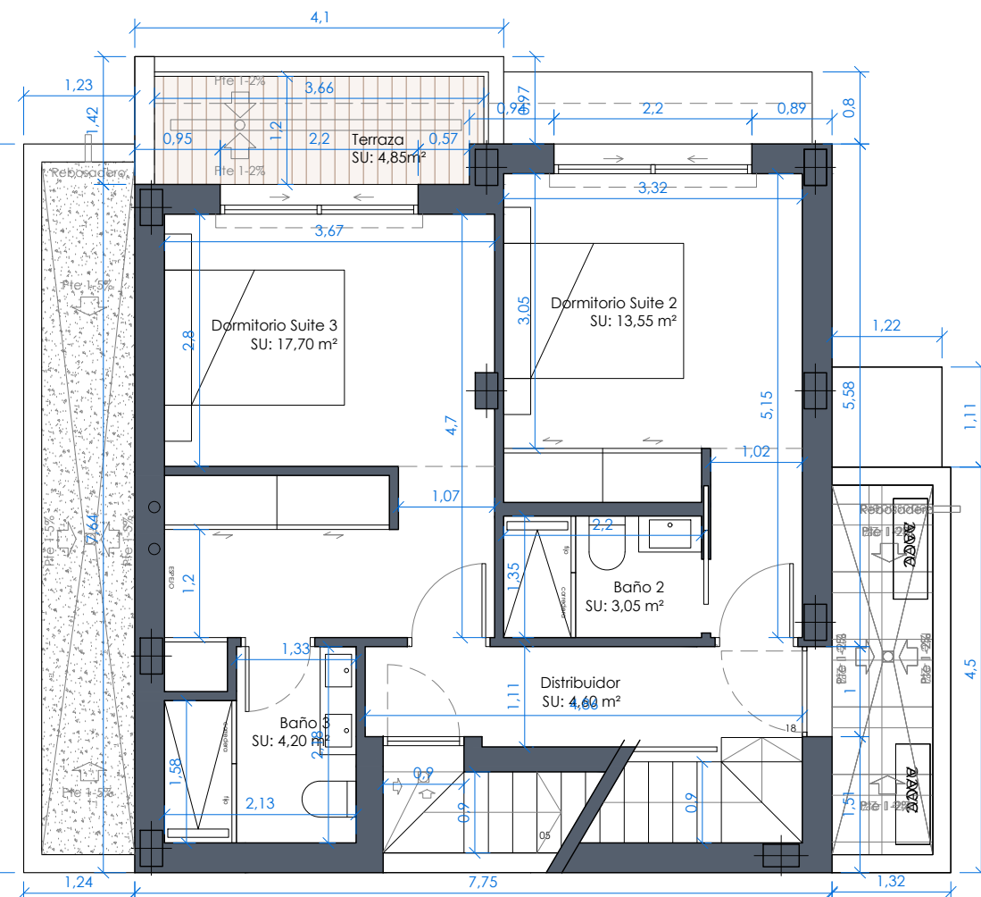
PLANTA PRIMERA
