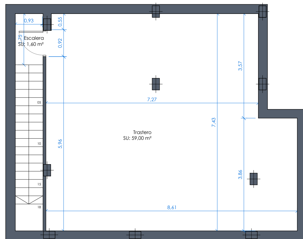
PLANTA SÓTANO
