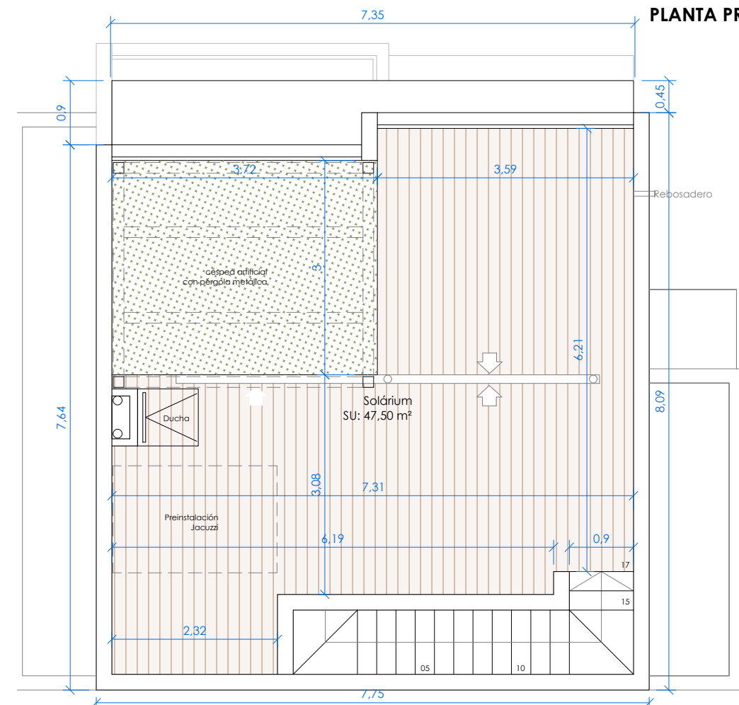
PLANTA CUBIERTA
