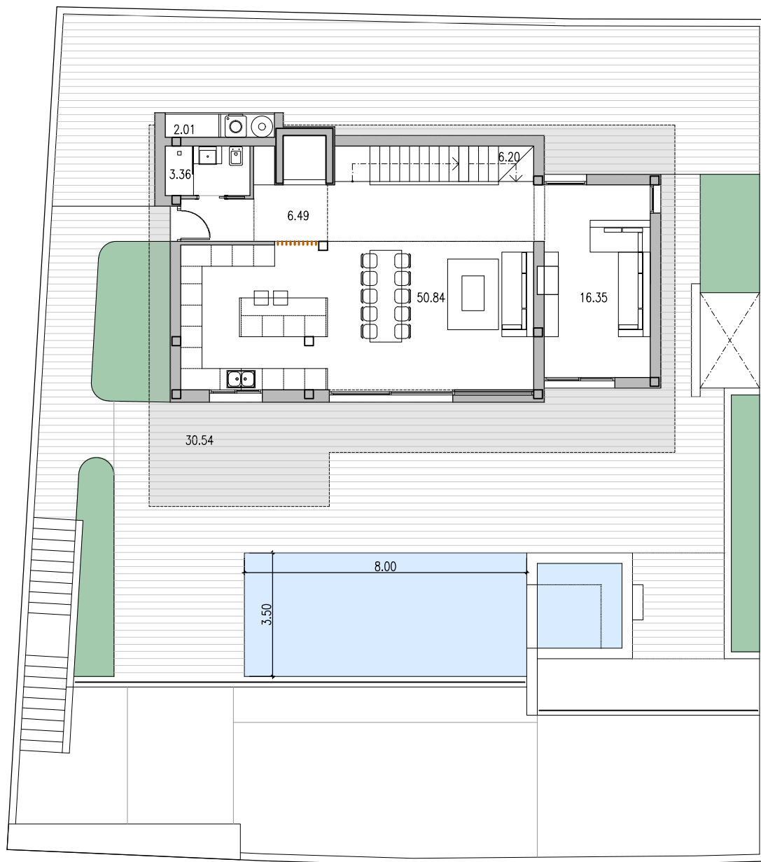
PLANTA BAJA
