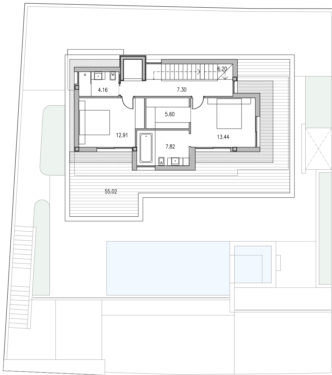
PLANTA PRIMERA
