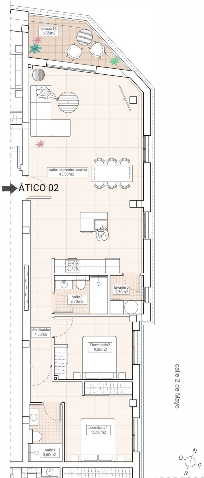
PLANTA ÁTICOS/ PENTHOUSE FLOOR
